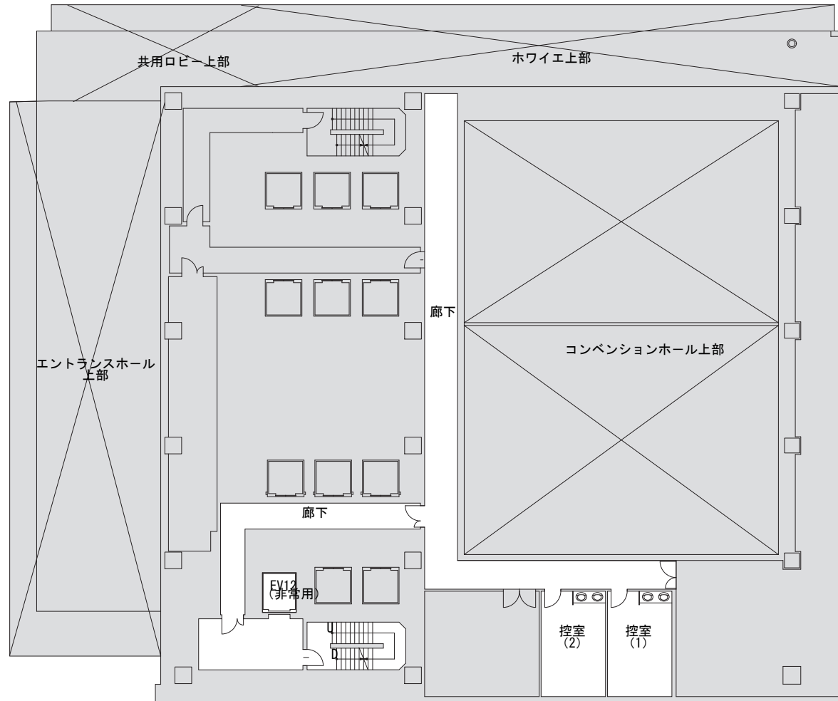
3階平面図
